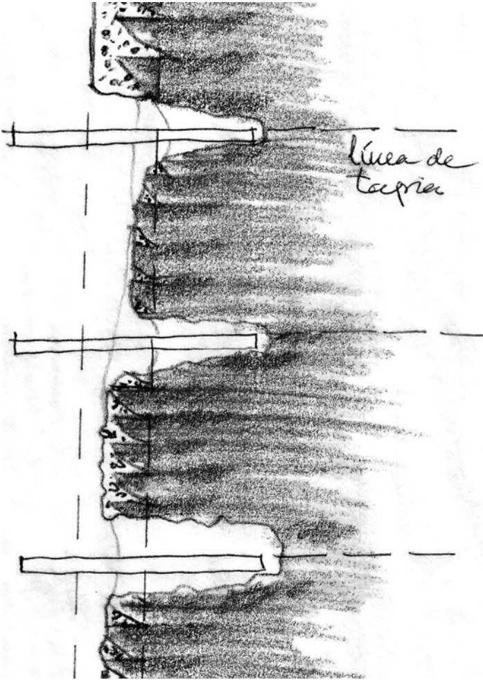
Croquis. Sección por los mechinales. (FJLM)
